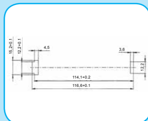
DIMA DI FORATURA 1,5 mm MAX.
