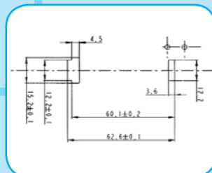
DIMA DI FORATURA
