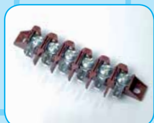
VEM 40R/6 Vo T 150°-450V-41A-6°
