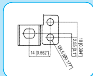
DIMA DI FORATURA 1,5 mm MAX.
