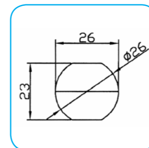
DIMA DI FORATURA 0,8/1,5 mm
