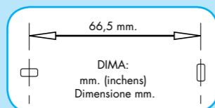
DIMA DI FORATURA 1,5 mm MAX.
